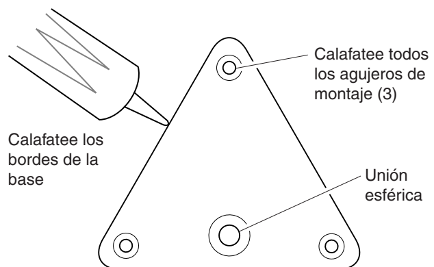
Tres agujeros de montaje para la base del panel solar
